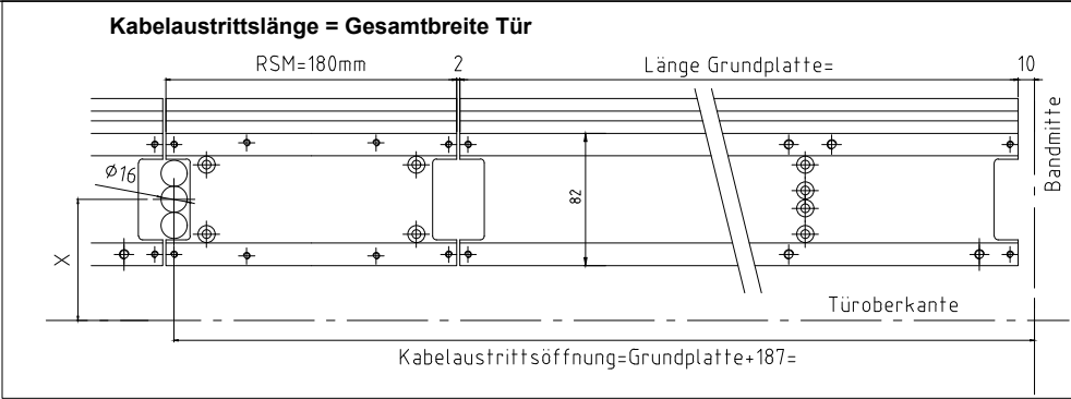
Ansicht Bandseite
