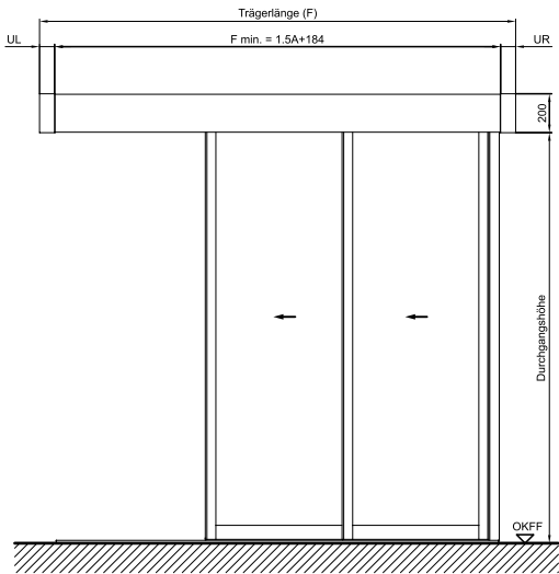
Grundriss
